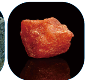
霞石
