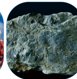
石灰岩
